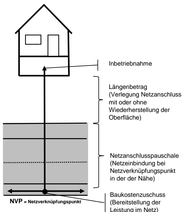
Abbildung 1: Zusammensetzung Standard-Netzanschluss ab Verteilleitung
