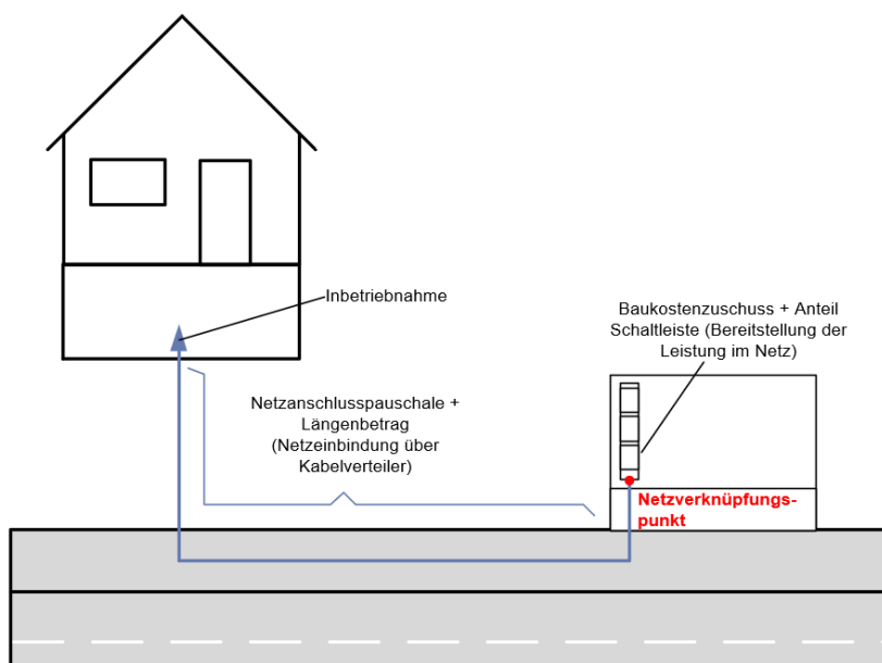
Abbildung 2: Zusammensetzung Standard-Netzanschluss ab Kabelverteilerschrank
